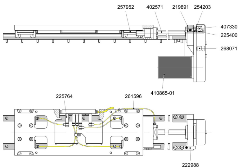
Schlitten-Planiereinheit RC
